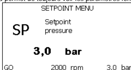
Image 15 Affichage d'un paramètre de menu
