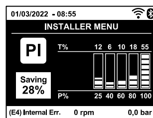
Obr. 17.2: Zobrazení sloupcového diagramu výkonu (3) (4)
