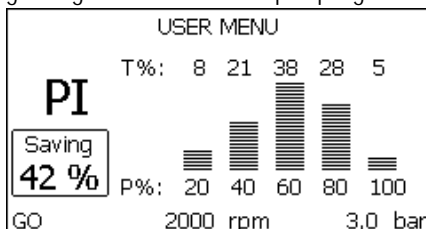
Afb. 17.1: weergave van het vermogenshistogram (2)
