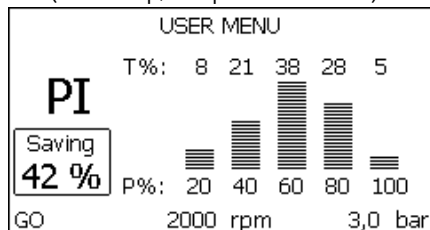
Figura 17.1: Vizualizarea histogramei de putere (2)
