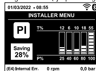
Afb. 17.2: weergave van het vermogenshistogram (3) (4)
