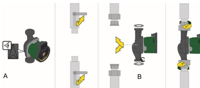
Малюнок 12: Монтаж EVOSTA2 SOL
